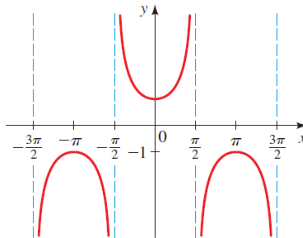
y = \sec x
