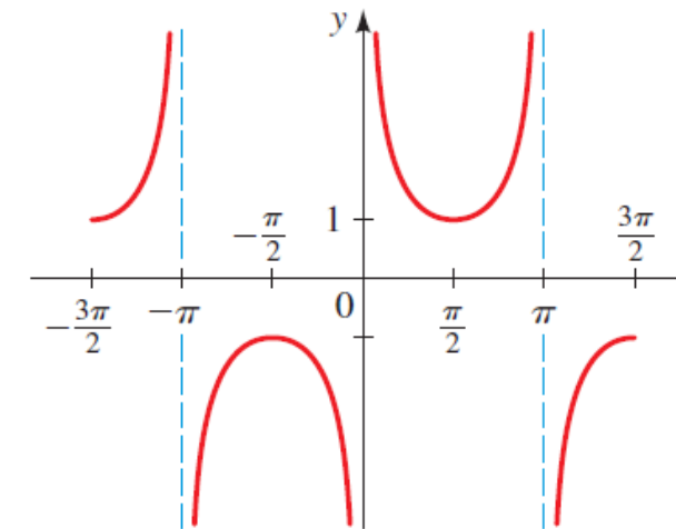
y = \csc x
